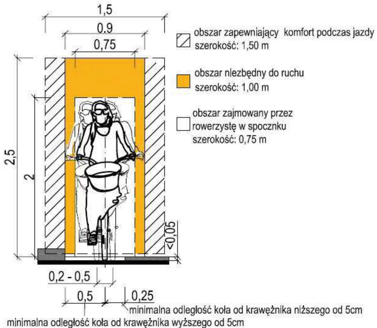
Rysunek 1. Skrajnia rowerowa
